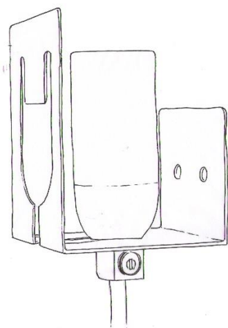
Lampeholder med 2-punktsophæng
